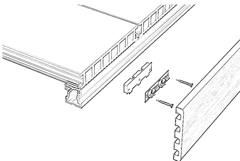
13. Montaż listwy wykończeniowej.
