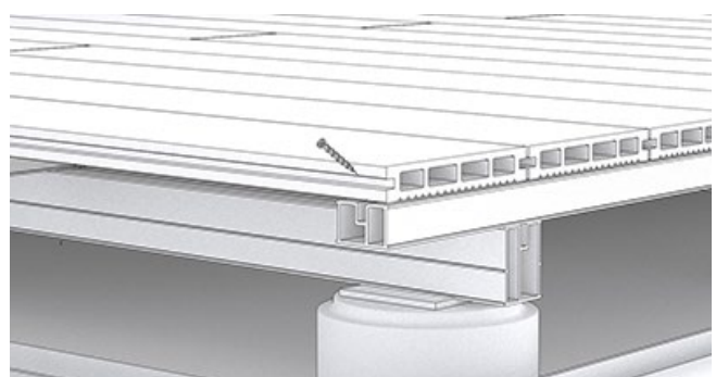
12. Przykręć uprzednio nawierconą deskę, zachowując kąt 45°.
