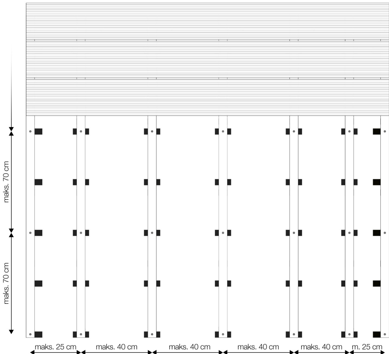
3. Podkonstrukcja na podłożu betonowym.
