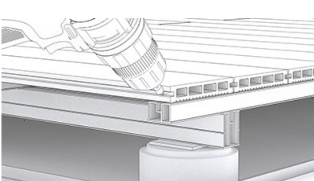
11. Nawierć ostatnią deskę pod kątem 45°.
