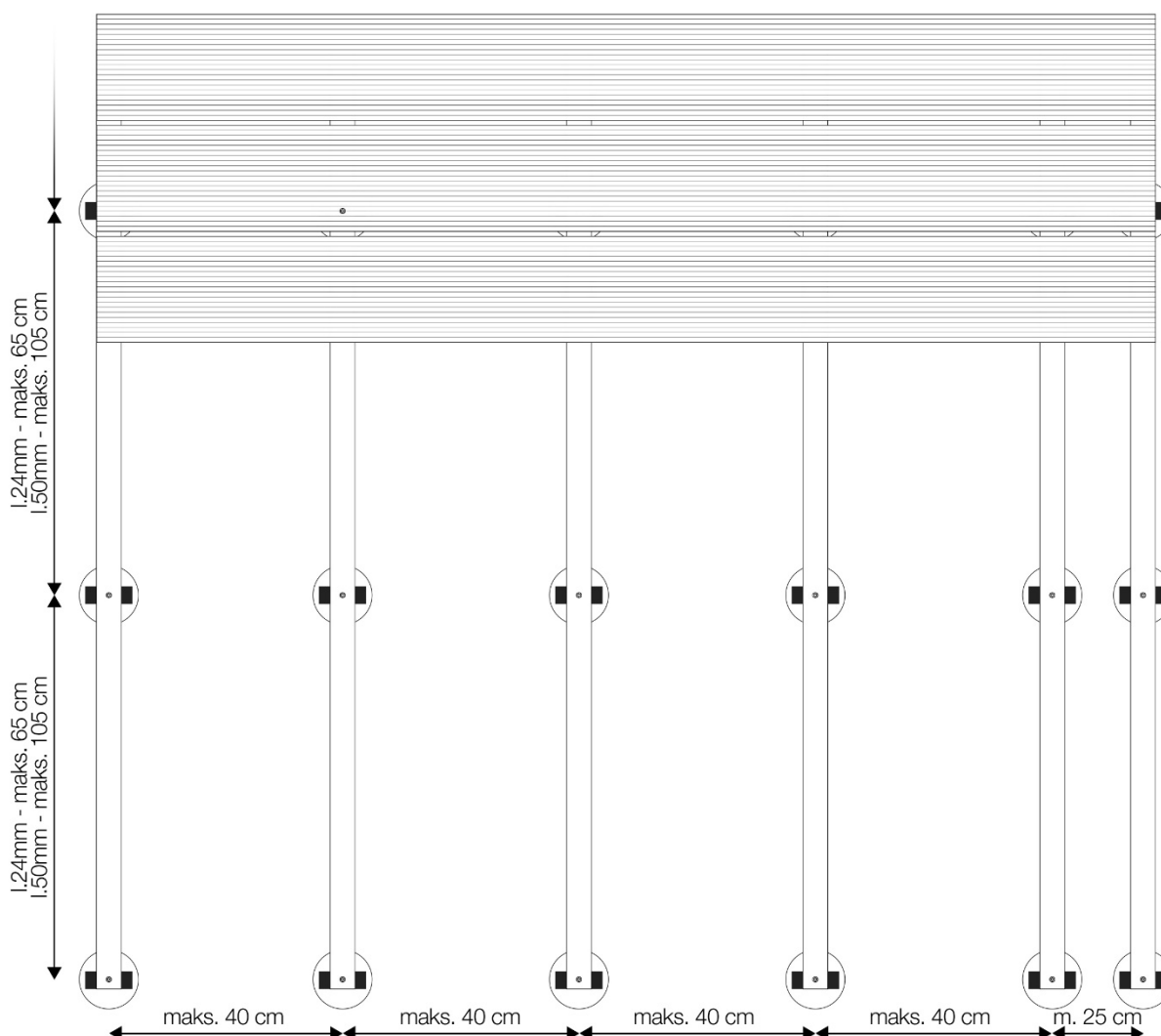
4. Podkonstrukcja na słupkach betonowych.
