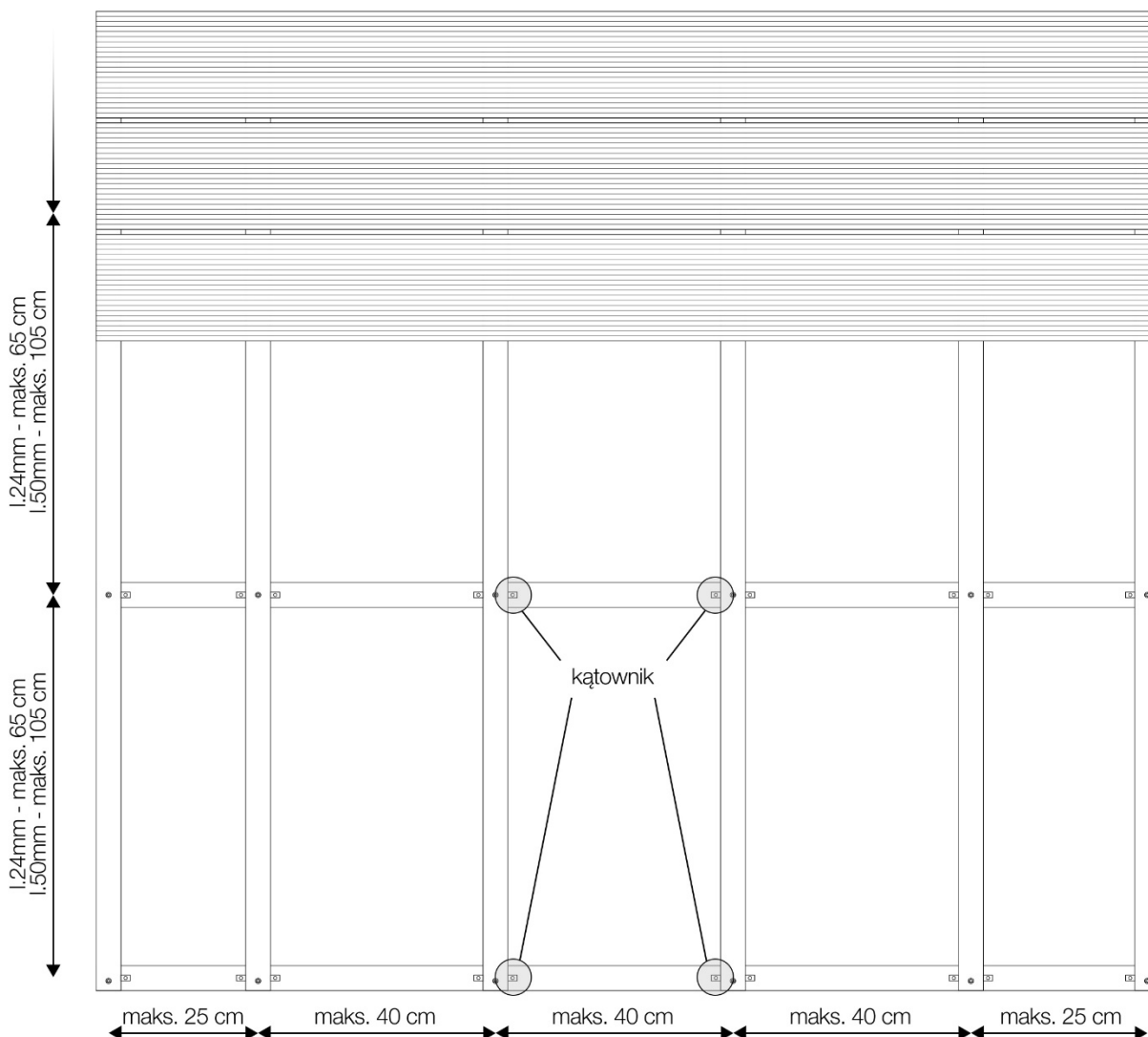
5. Podkonstrukcja Kratownica – podwójne legarowanie.
