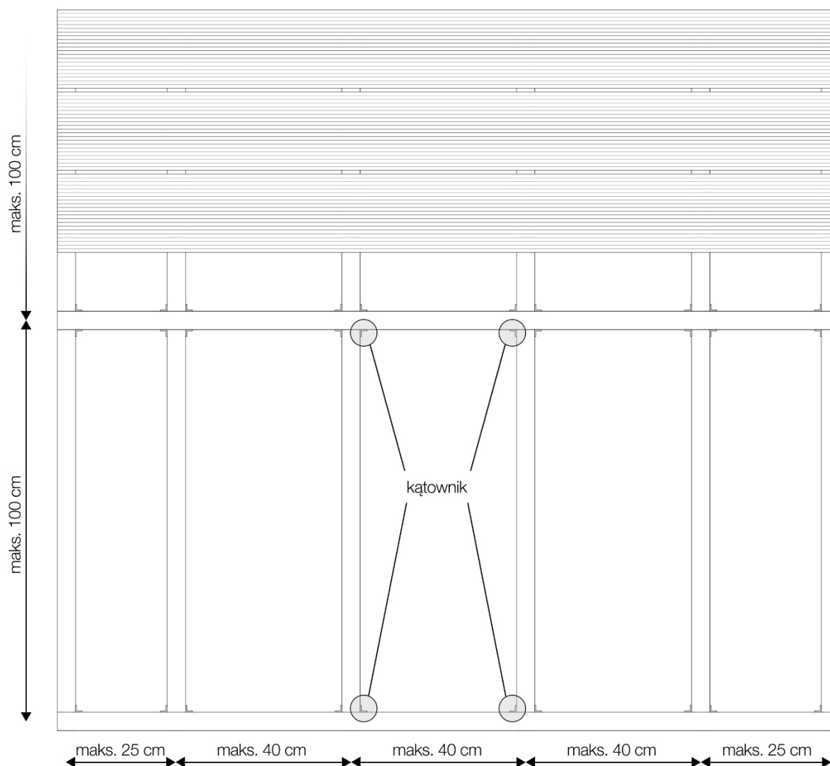
6. Podkonstrukcja Rama pojedyncza z żebrami usztywniającymi.
